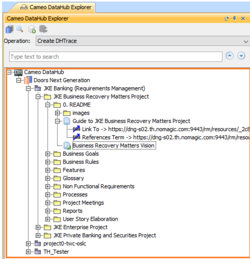
The DataHub tree.
