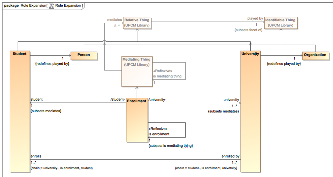
Example of the «Role» Pattern Expansion
